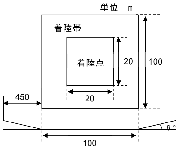
d-1 大型機 <CH-47> の場合《標準》
