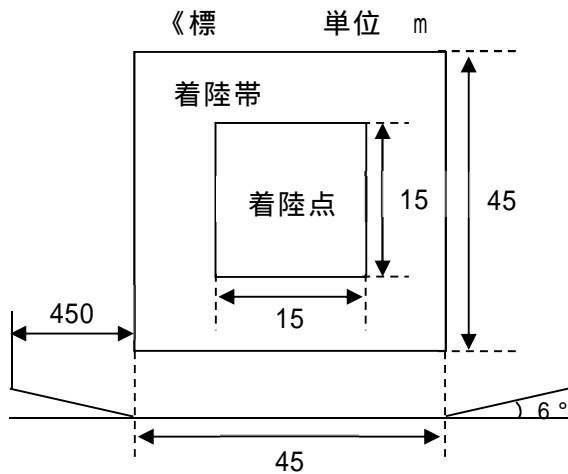
c-1 大型機 <V-107及びUH-60J> の場合
