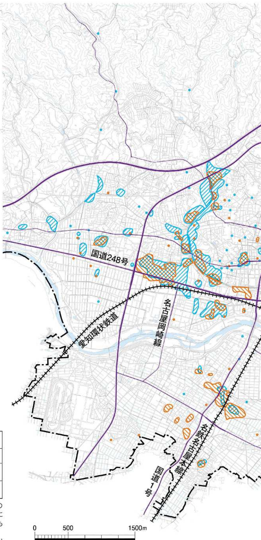
時間雨量図(平成20年8月末豪雨) (平成20年8月28～30日)
